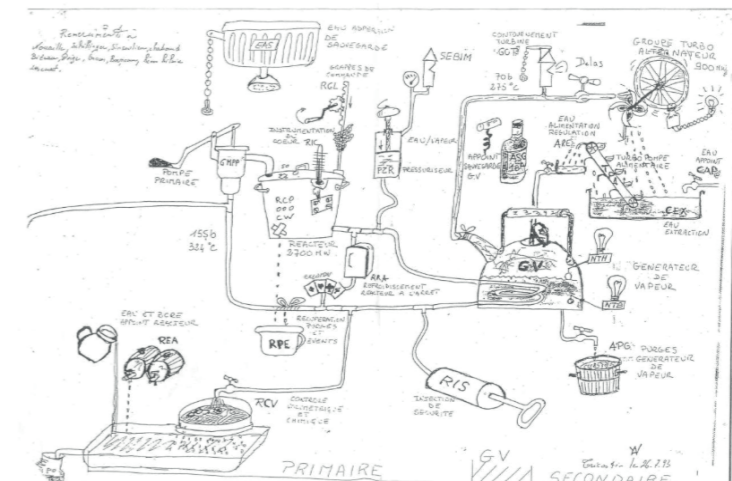
Vulgarisation du fonctionnement d'une centrale par Framatome (1993)
